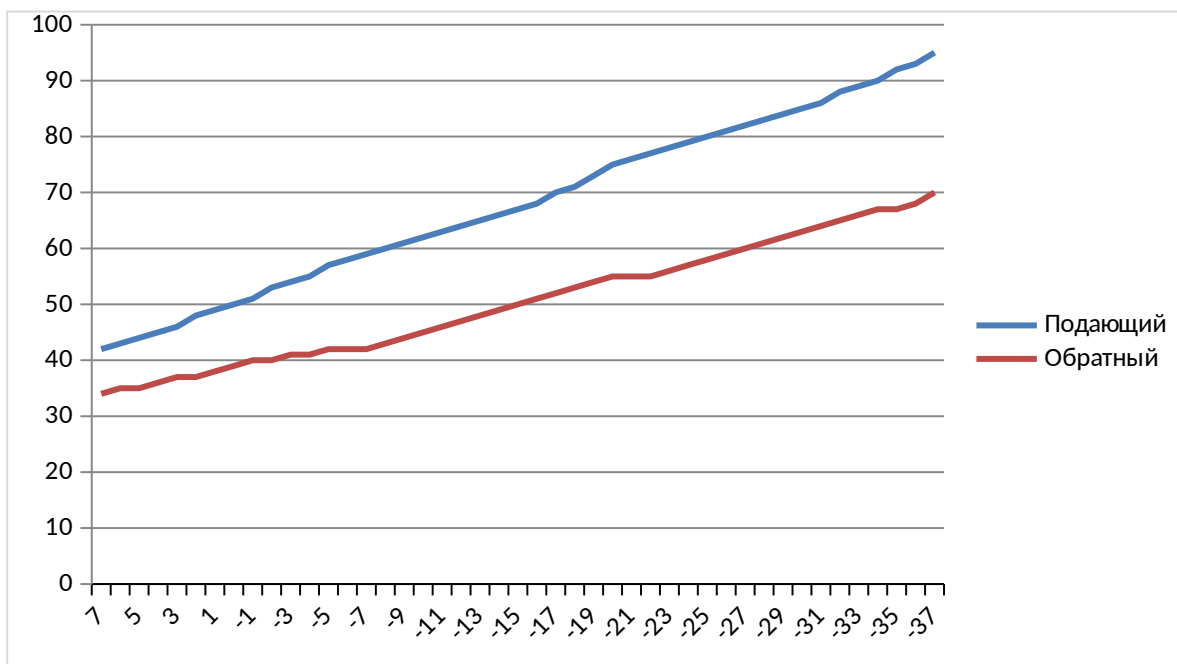
Температурный график
