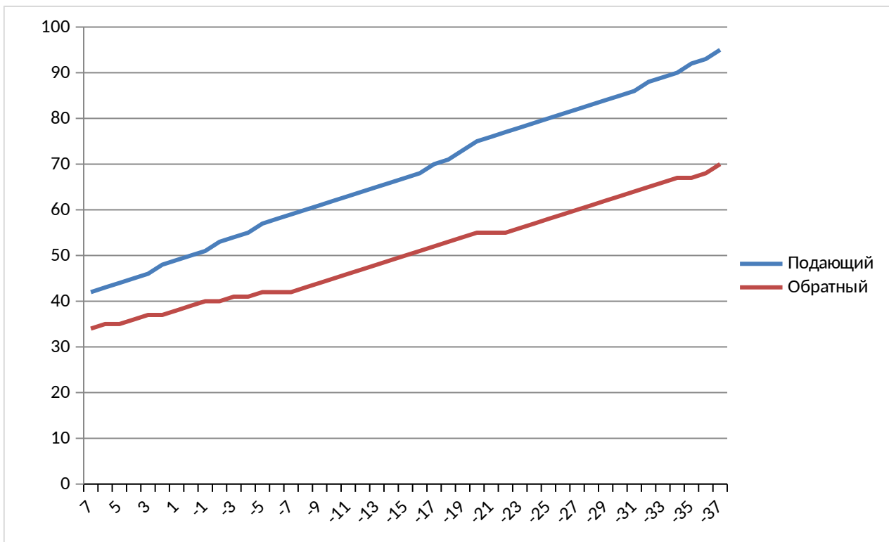
Температурный график
